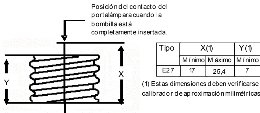
Figura 16. Posición de la camisa roscada del portalámpara [mm]
