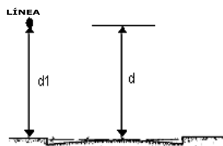
Figura 6. Distancias "d" y "d1" en cruces y recorridos de vías
