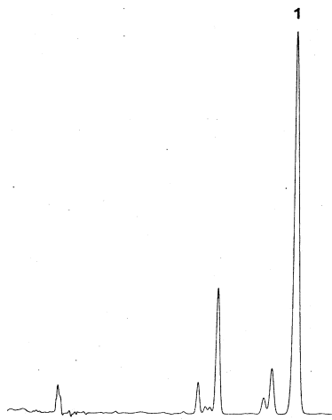
图1 咪鲜胺乳油的高效液相色谱图
