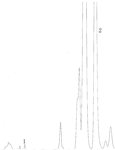
图2 咪鲜胺乳油中 2, 4, 6-三氯苯酚的高效液相色谱图
